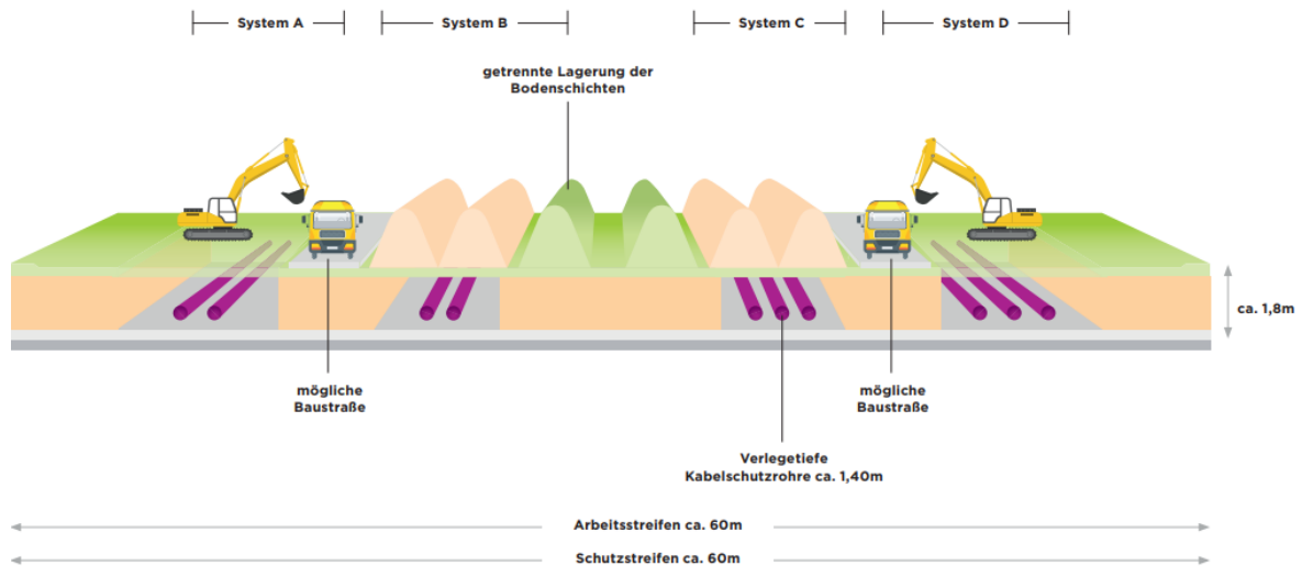
KORRIDOR B REGELGRABENPROFIL STAMMSTRECKE
