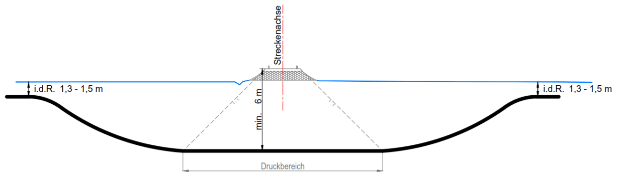
Abbildung 19: Beispiel Bahnkreuzung mit HDD-Verfahren
