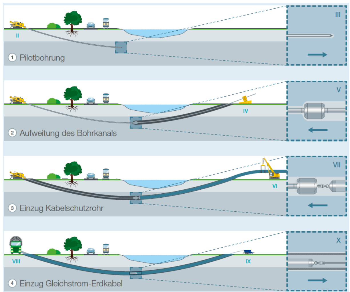
Abbildung 20: Beispiel HDD-Verfahren
