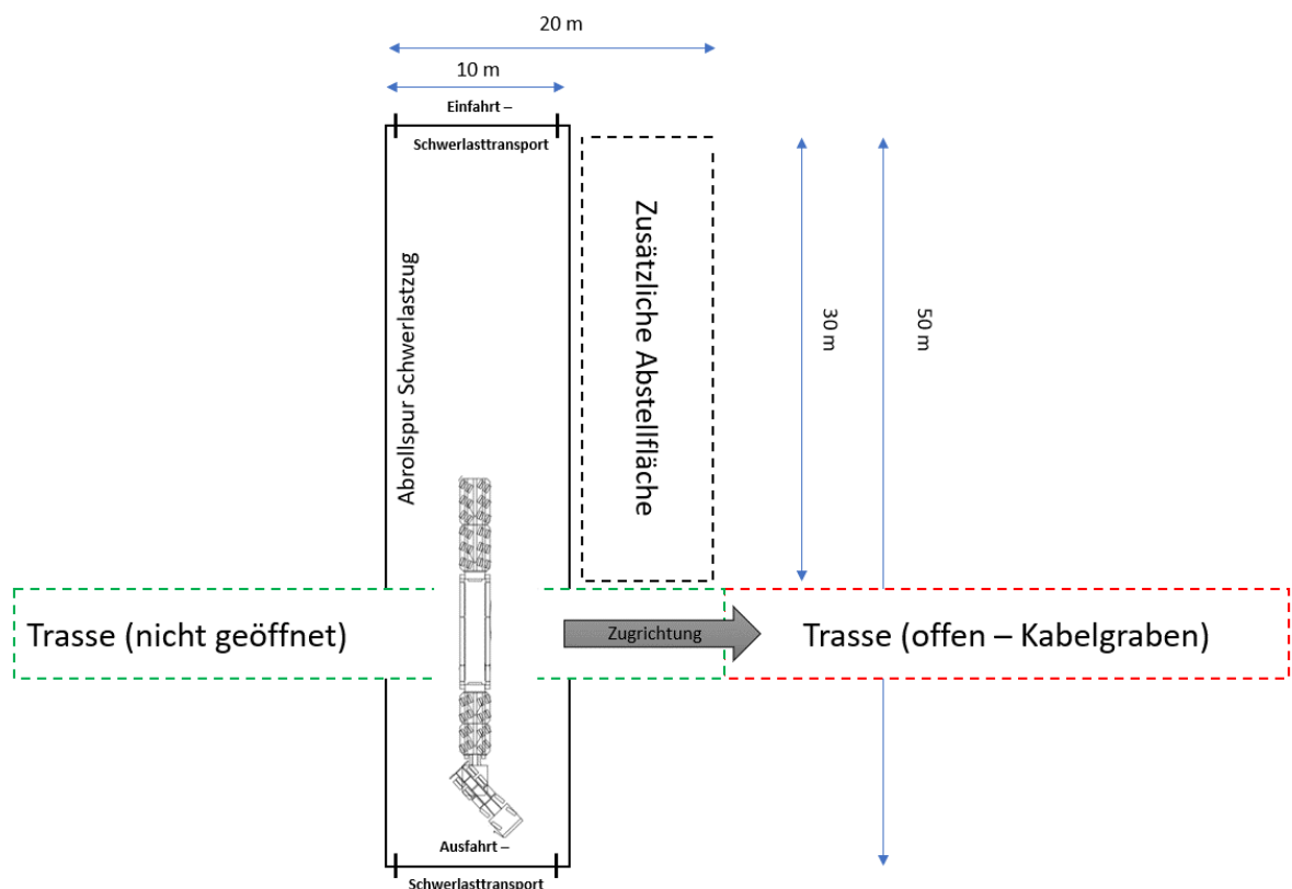
Abbildung 11: Beispiel Abspulung über Kabelgraben
