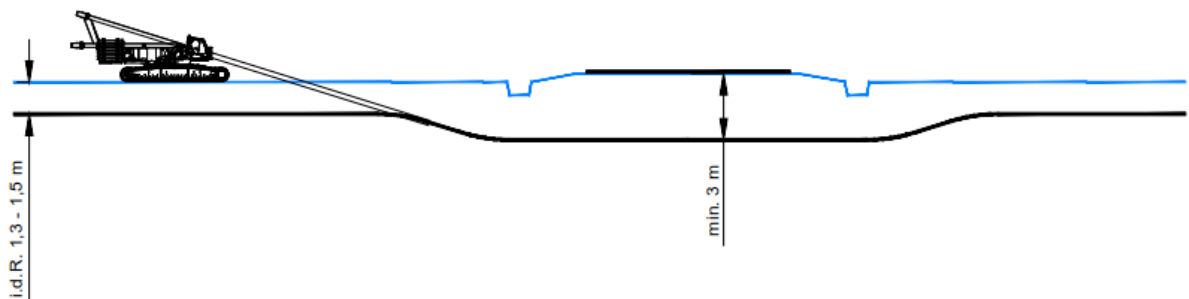
Abbildung 21: Typische Mindestüberdeckungen bei HDD-Querungen
