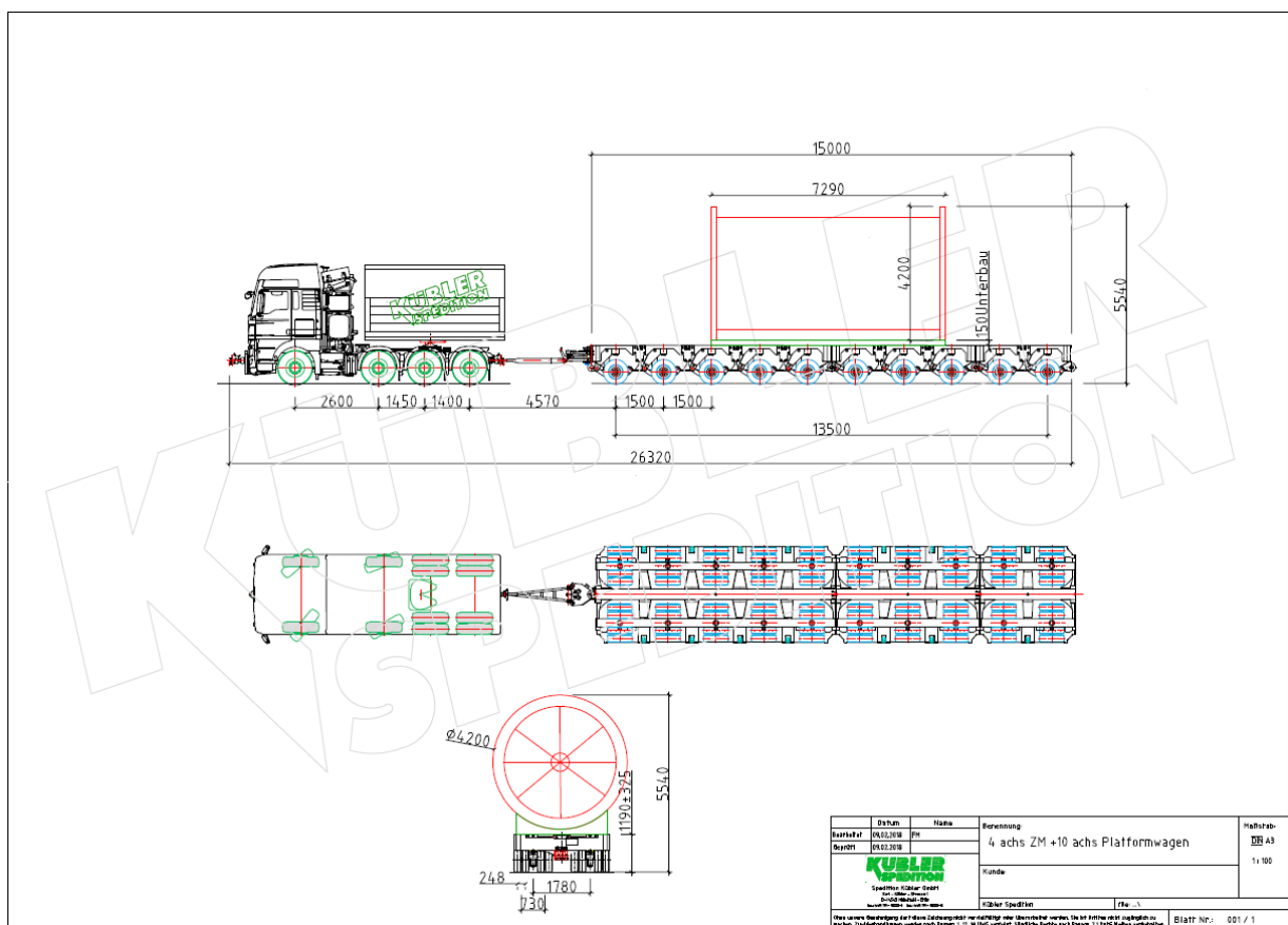
Abbildung 10: Skizze Plateau-Fahrzeug
