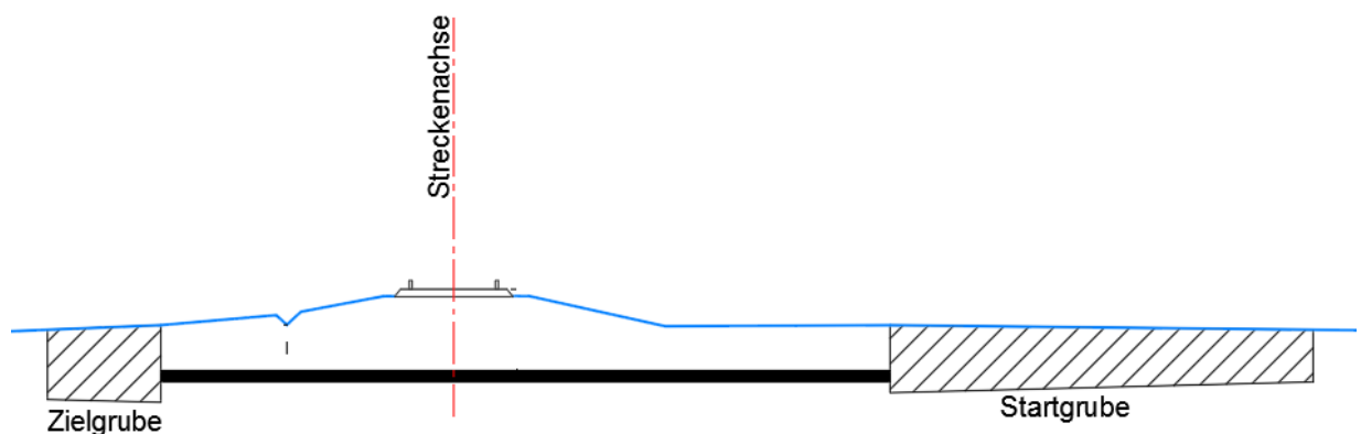
Abbildung 18 Schematische Skizze Rohrvortriebsverfahren
