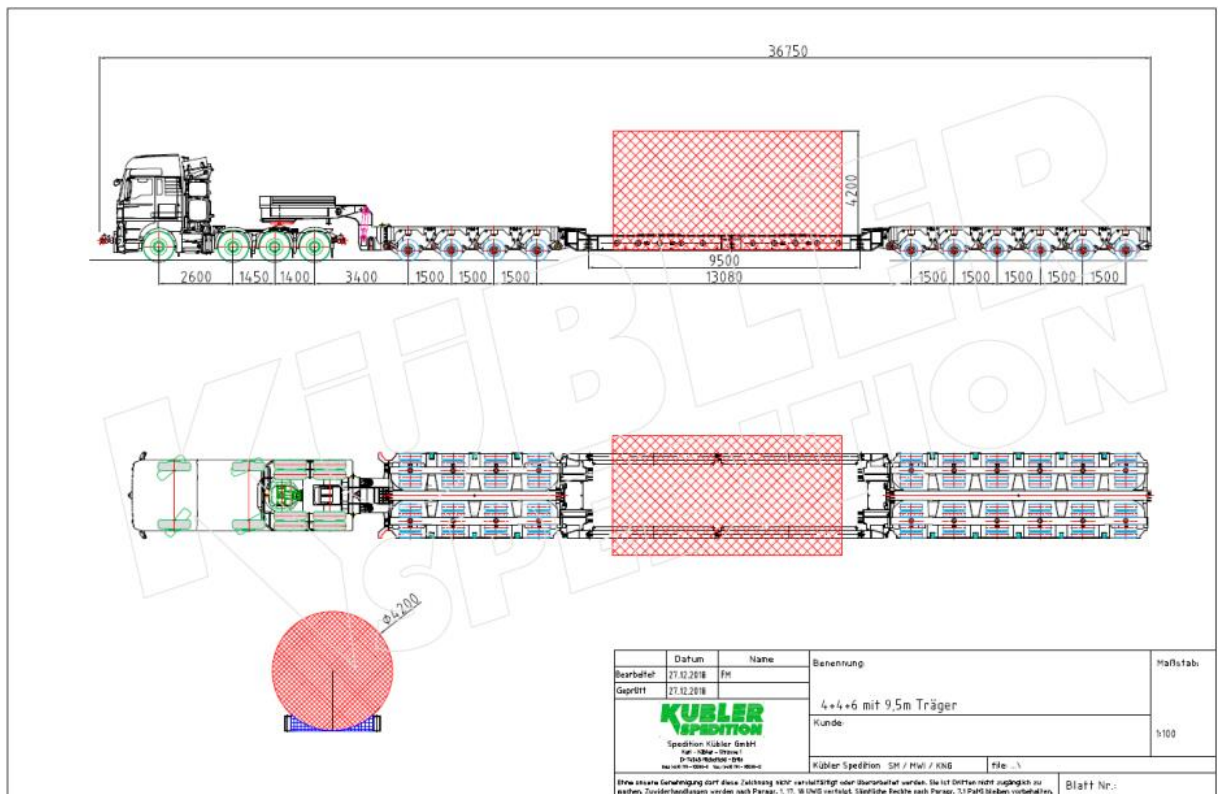
Abbildung 9: Skizze Kesselbrücke
