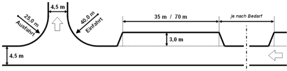
Abbildung 12: Skizze einer Baustraße
